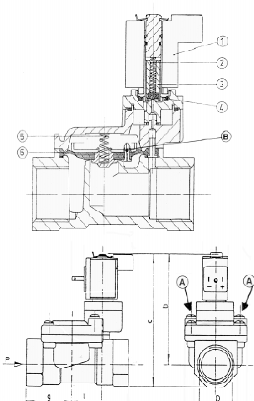
ELETTROVALVOLA
